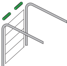
■ Наклонный высокий тип монтажа с верхним расположением вала
